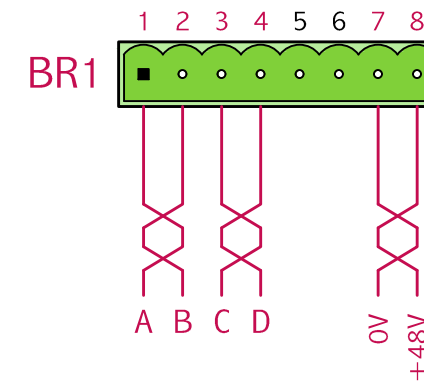
RACCORDEMENT UTILISATEUR
